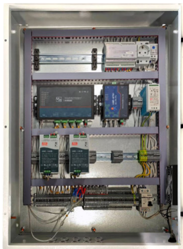
Декаст Шкаф АСКУВТ 8RS-LTE
