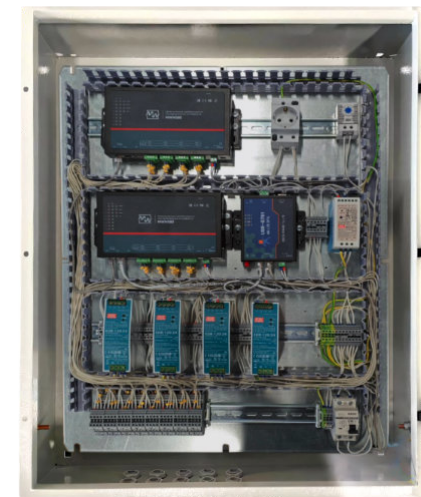
Декаст Шкаф АСКУВТ 16RS-LTE
